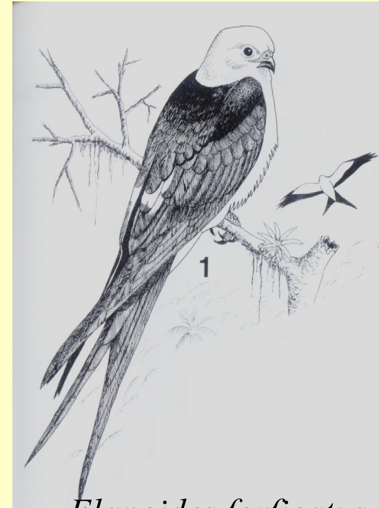
Elanoides forficatus
